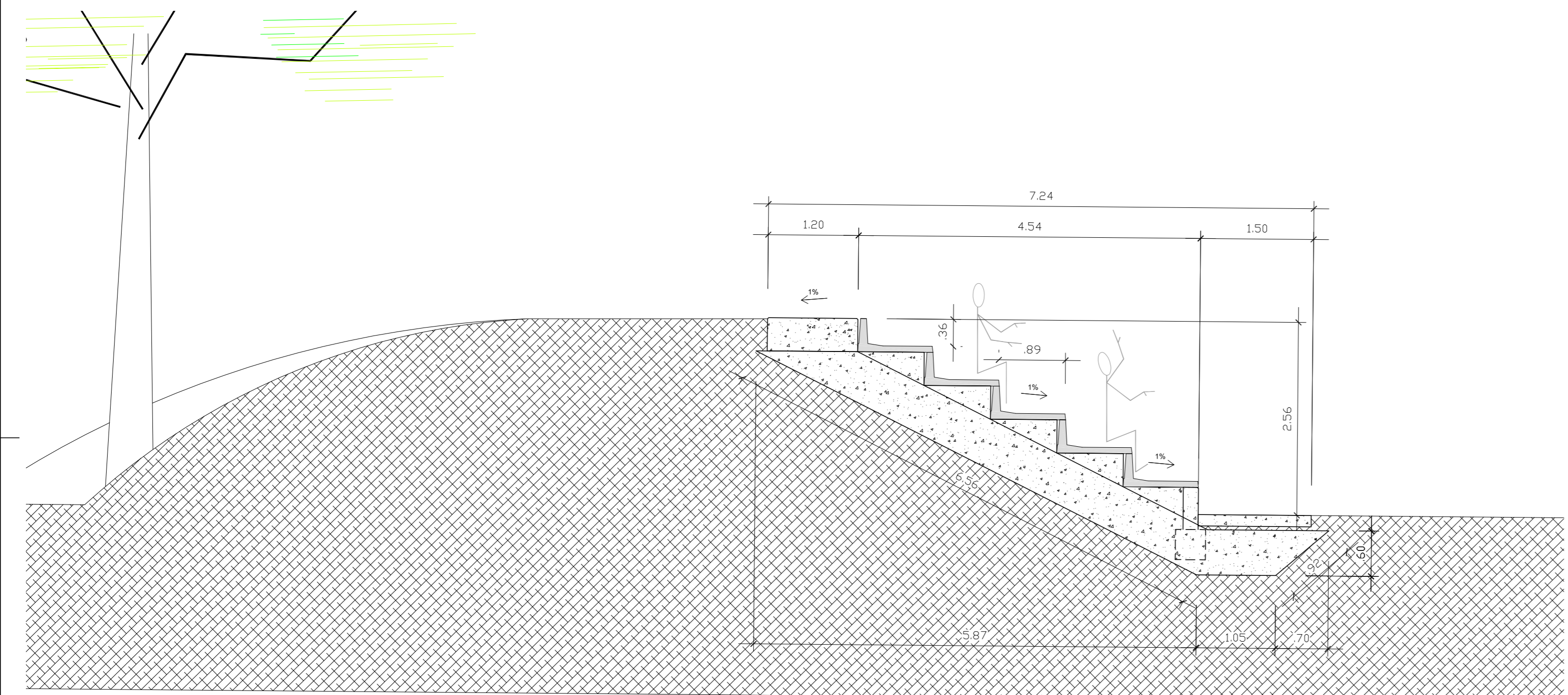
SECCIÓ A-A'
