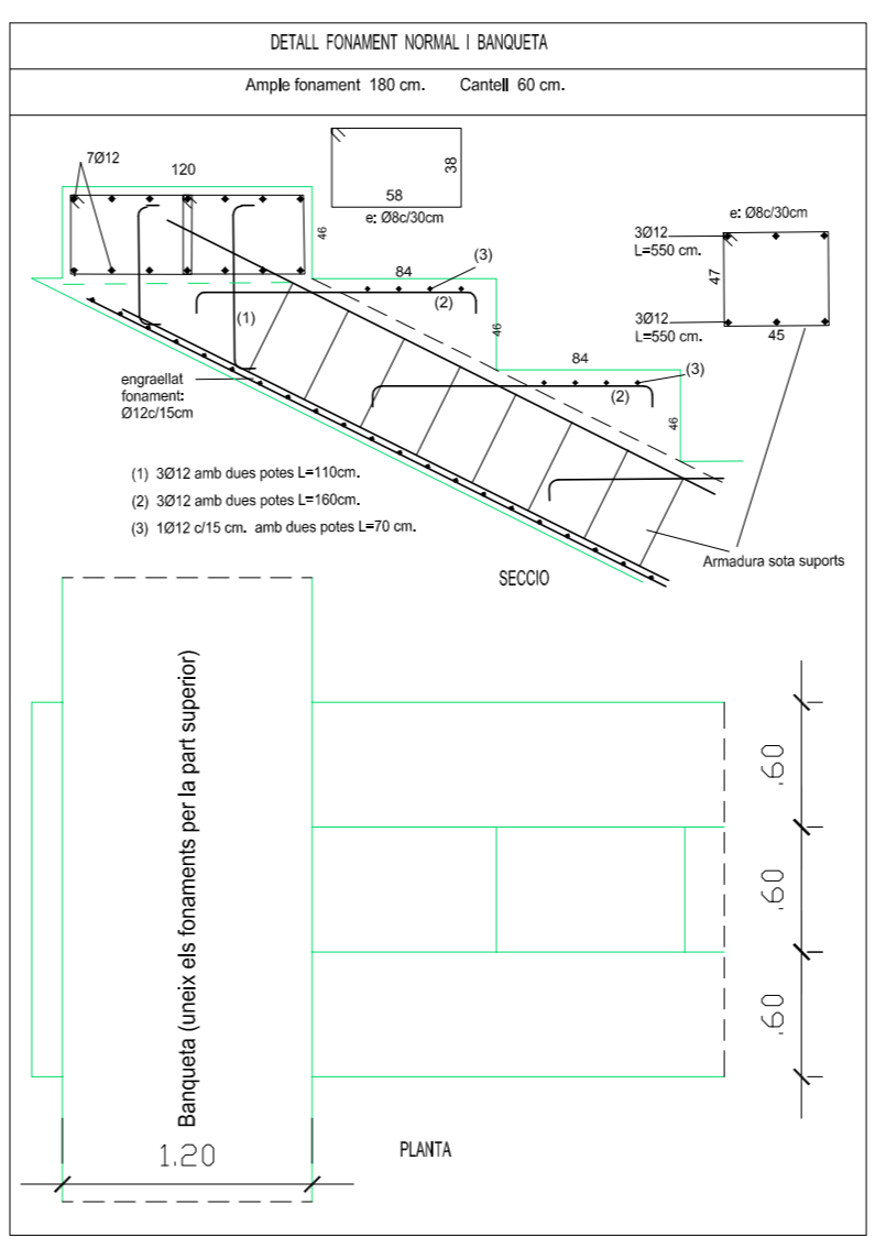
DETAILS FONAMENTS
